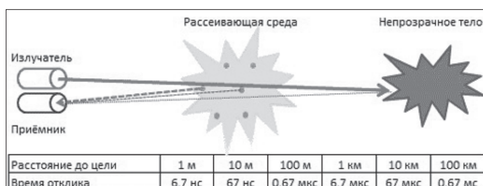
Схема на принципа на действие на новия руски детектор на взривни вещества, наречен ЛИДАР (от английското съкращение LIDAR - Light Identification, Detection and Ranging)
