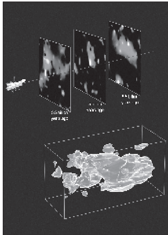
Учените така представят разпределението на тъмната материя: Преди 3,5 млрд., 5 млрд. и 6,5 млрд. години
