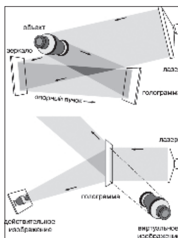
Опростена схема на холографичния скенер
