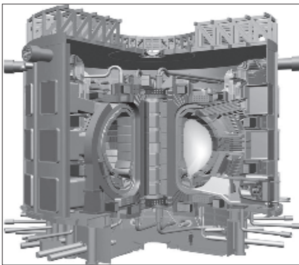
Конструкция на реактора ITER, чието изграждане (във Франция) вече е в ход. Проектът трябва да бъде завършен през 2018 г. Мощността на реактора трябва да е не по-малко от 500 МВт. На чертежа долу е нарисувана човешка фигура, която дава представа за големината на ITER
