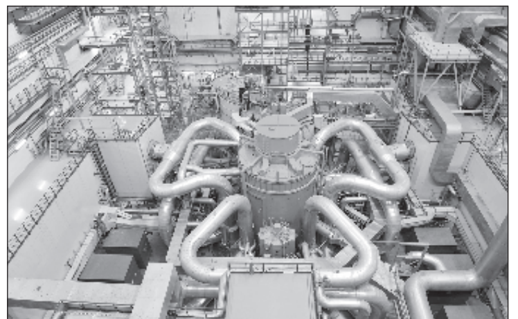
Реактор на бързи неутрони "БН-800"
