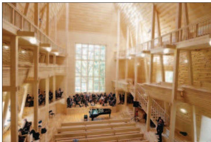
В 2017-м в курортном поселке Репино, рядом с Финским заливом, открылся концертный зал, построенный на средства Гергиева. Авторами проекта выступили архитектор и реставратор Ксавье Фабр и инженер акустического проектирования Ясухиса Тойота
